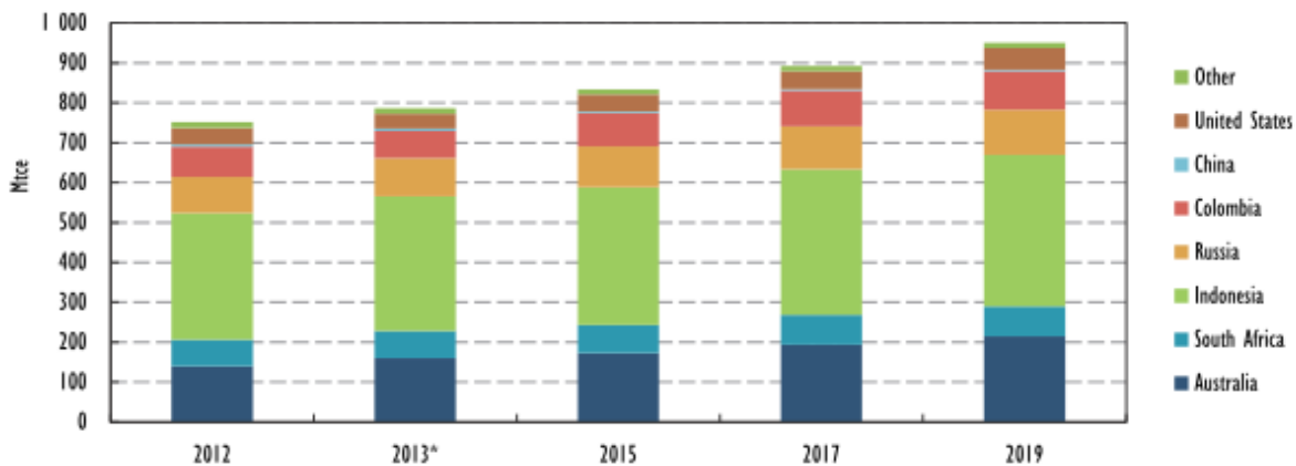
(b) Berechnungen mit dem ewi-Modell TIMCO zeigen zunehmende seewärtige Steinkohlexporte 2013-19
