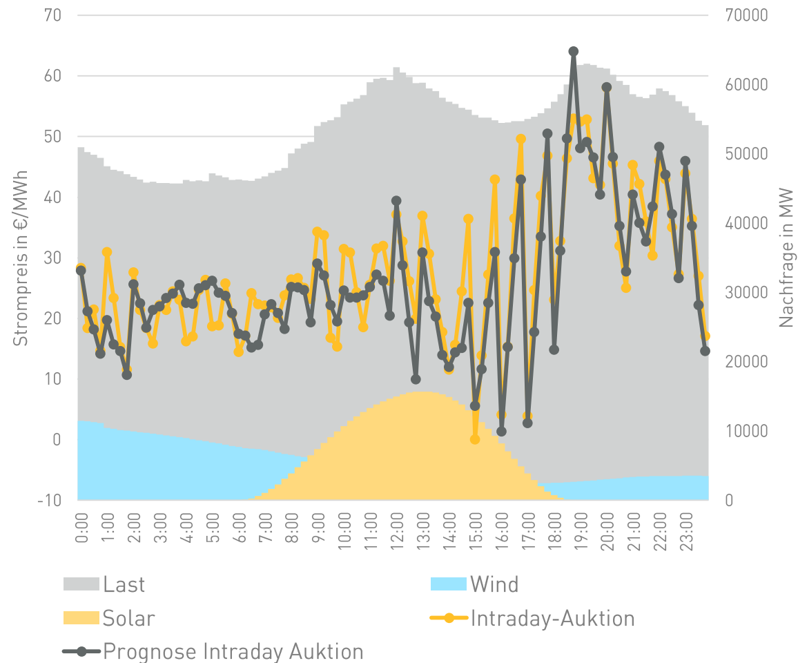
(a) Prognose der Viertelstundenauktionsergebnisse auf Basis von Profilen der erneuerbaren Energien sowie Nachfrage und knappem Angebot aufgrund von Flexibilitätsbeschränkungen
