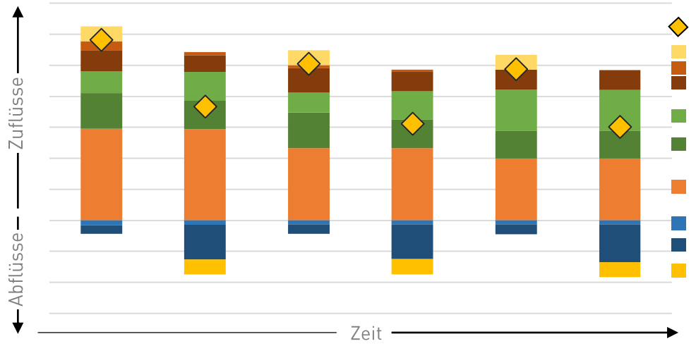
(a) Beispielhafter Modelloutput: Länderweise Gasbilanz 2015-2017
